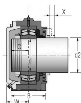
Execução Cega
