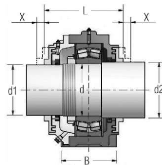
Execução Passante
