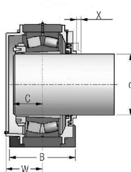
Execução Cega
