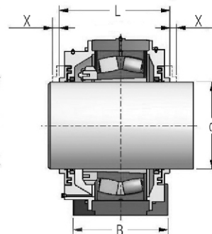
Execução Passante
